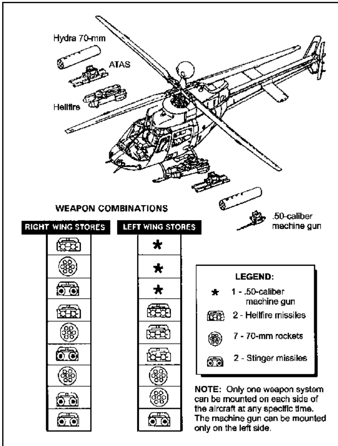
Figure 6-7. OH-58D(I) Kiowa Warrior.
